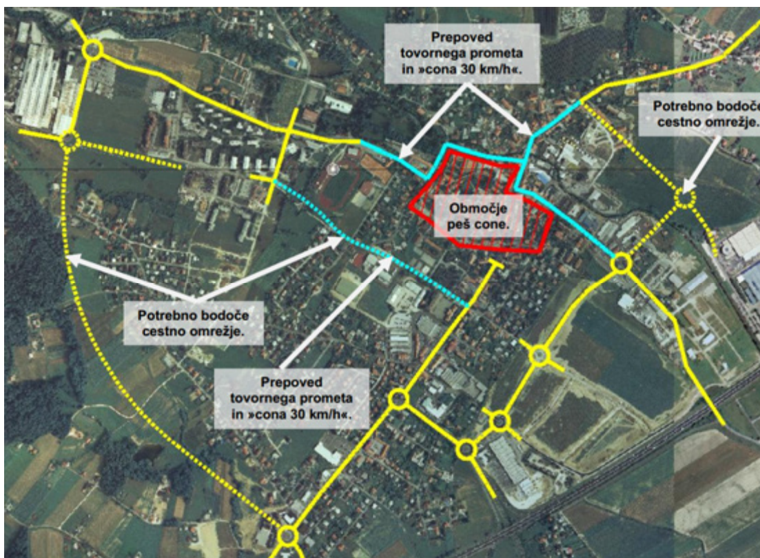
Slika 23: Predlog prometne ureditve mesta ob vzpostavitvi »pešcon« v mestnem jedru Vir: Novelacija prometne študije širšega območja mesta Slovenska Bistrica, TRASA, d. o. o., 2016
